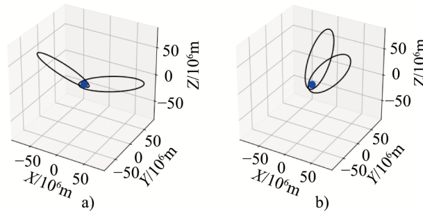
注: a) 优化前轨道结构图; b) 优化后轨道结构图。优化前的性能指数 S 为 15.960, 经优化后降至 11.231。 S 值越小, 轨道构型越优。
