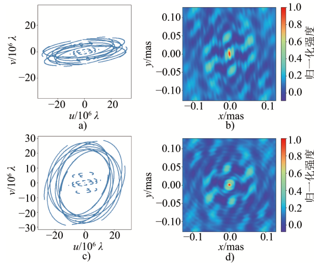
注：在 uv 覆盖分布方面：a) 为 M87 源优化前的 uv 覆盖，c) 为 M87 优化后的 uv 覆盖。优化后配置提升了空间频率采样的均匀性，并扩展了基线覆盖范围。在合成波束特性方面：b) 为 M87 优化前的波束图，d) 为 M87 优化后的波束图。优化后的波束表现出更接近圆形的特性，且旁瓣水平有所降低（旁主瓣比减小）。轨道优化前后的对比参数在表 2 中列出。
