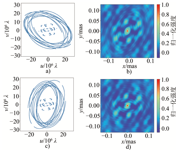
注: 在 uv 覆盖分布方面: a) 为银河系中心 (Sgr A*) 优化前的 uv 覆盖, c) 为银河系中心 (Sgr A*) 优化后的 uv 覆盖。优化后的空间频率采样均匀性有所提高, 基线覆盖范围有所扩展。在合成波束特性方面: b) 为银河系中心 (Sgr A*) 优化前的波束图, d) 为银河系中心 (Sgr A*) 优化后的波束图。优化后的波束表现出更接近圆形的特性, 且旁瓣水平有所降低 (旁主瓣比减小)。轨道优化前后的对比参数在表 2 中列出。
