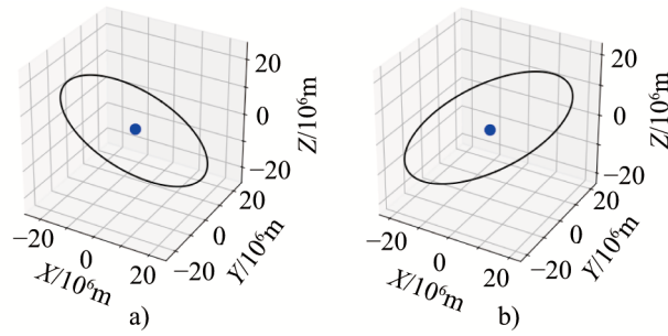
注：a) 优化前轨道结构图；b) 优化后轨道结构图。优化前的性能 S 指数为 1.870，经优化后降至 1.697。
