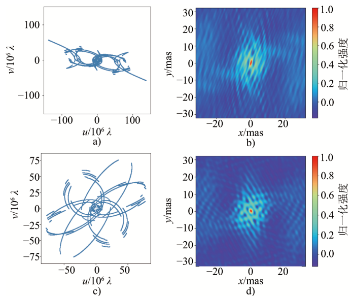
图 5 在 300 MHz 观测频率下的第二个目标源优化前后 uv 覆盖和合成波束对比结果
