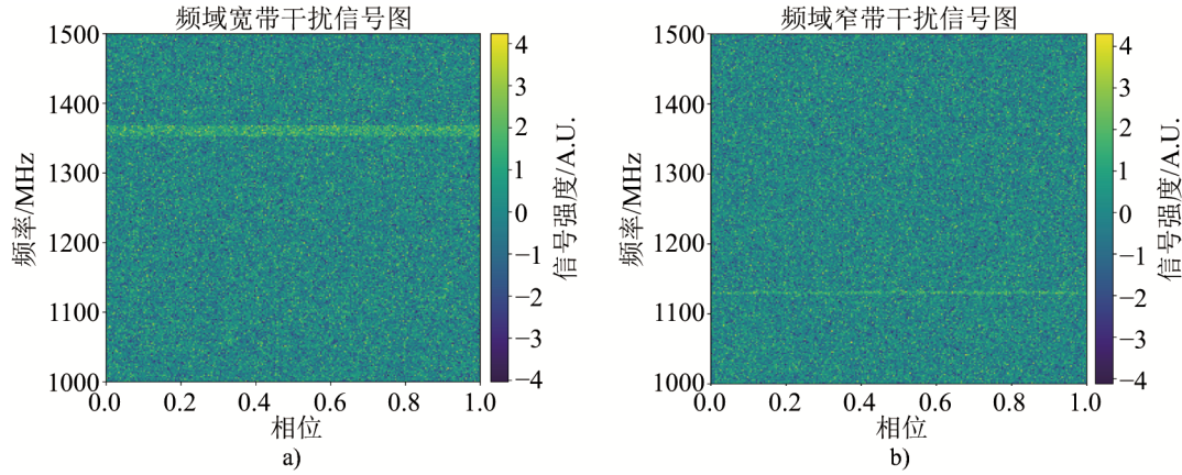
图 1 脉冲星候选体样本模拟中的频域宽带干扰和频域窄带干扰
