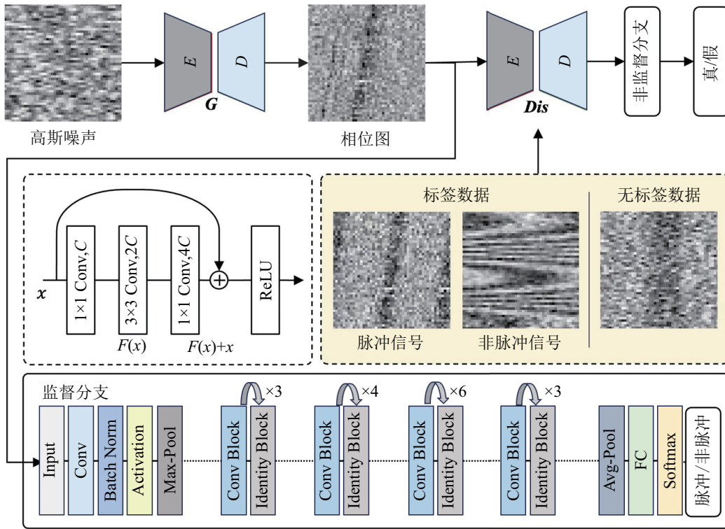
图 6 改进模型 (ResGAN) 网络架构
