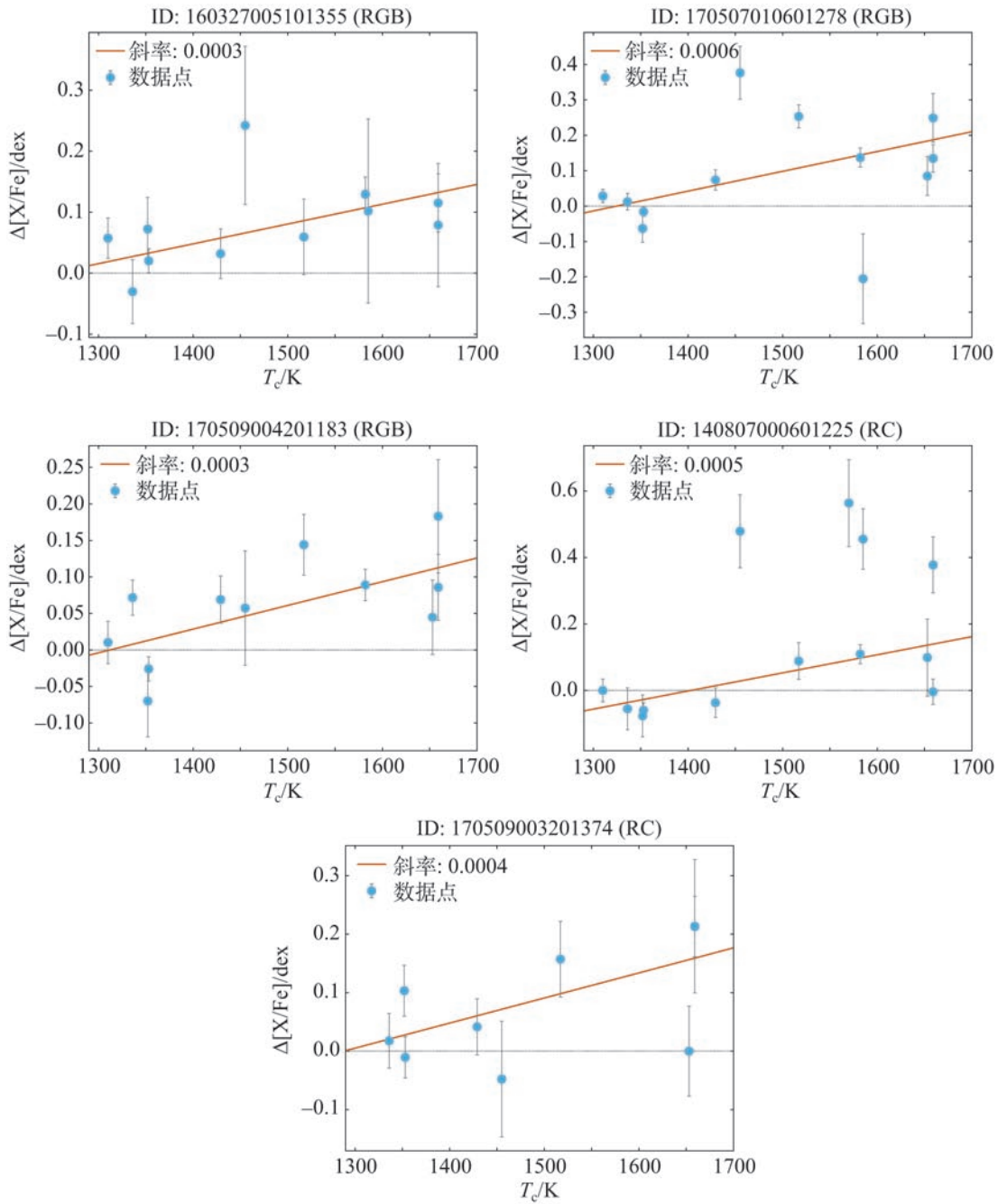
图 3 5 颗吞噬迹象候选体样本的 \Delta[X/Fe] 与 T_c 关系
