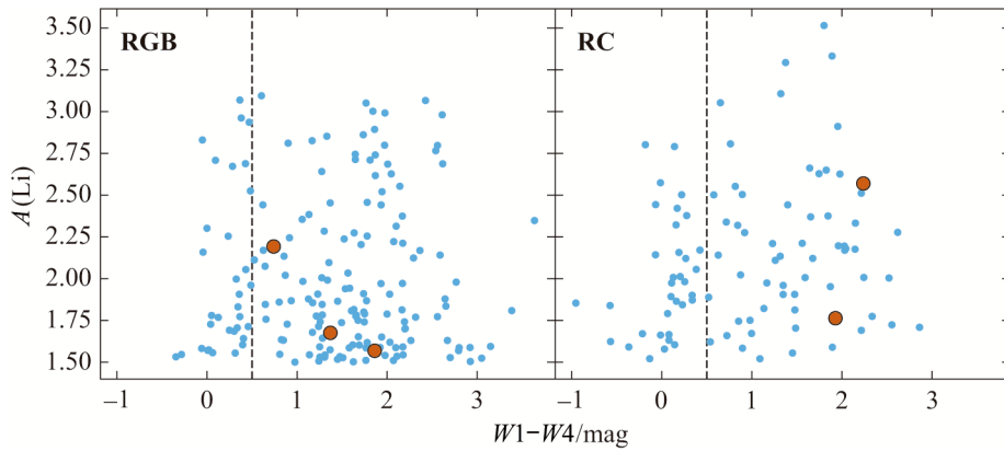
图 4 271 颗富锂巨星的红外超 W1 - W4 与锂丰度 A(\text{Li}) 的关系
