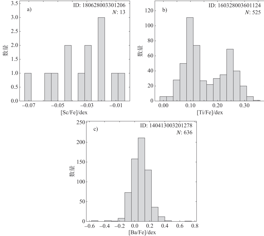
图 2 富锂巨星的孪生星样本元素分布
