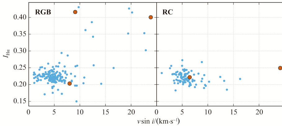
图 6 271 个富锂巨星的磁活动指标 I_{H\alpha} 与投影自转速度 v \sin i 的关系
