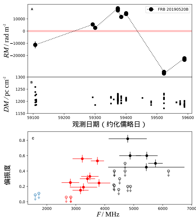
图 6 FRB 20190520B 的 RM、DM 与时间的关系以及偏振度与频率的关系图。A: RM 随时间的变化; B: DM 随时间的变化; C: 偏振度与频率的关系 [22] 。
