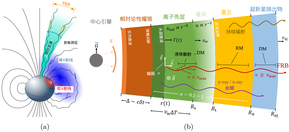
图 3 (a) 快速射电暴的类脉冲星模型 [44] ; (b) 快速射电暴的类伽马射线暴模型 [49] 。
