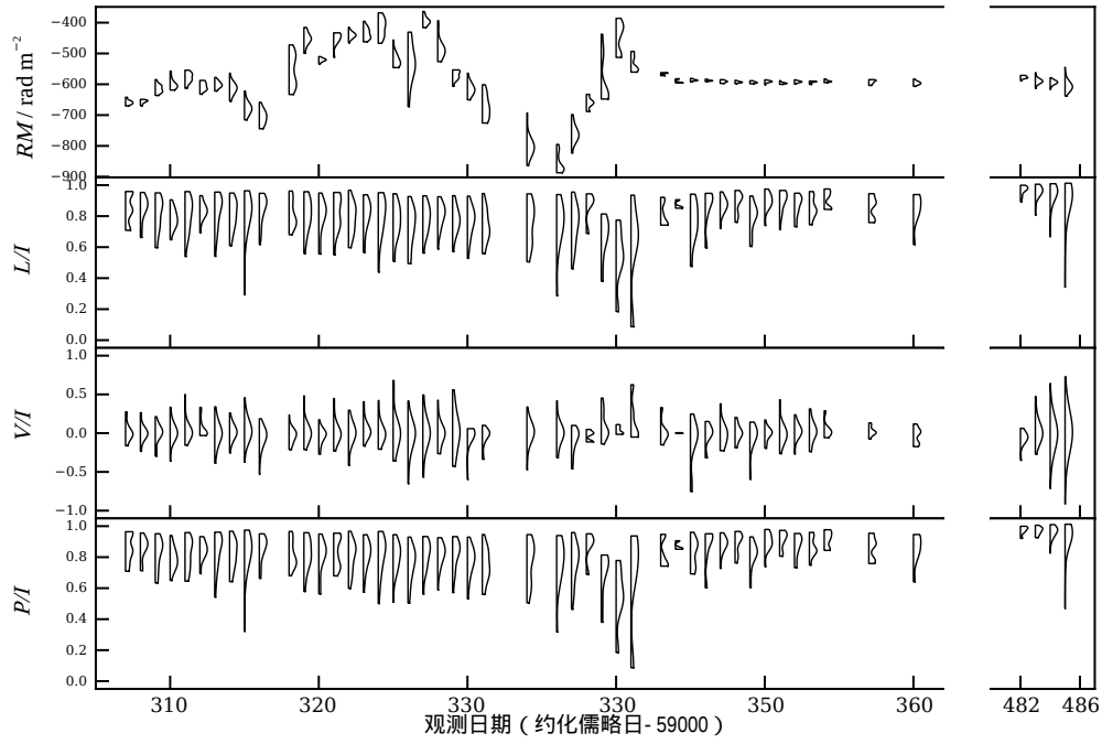
图 7 FRB 20201124A 的 RM、 L/I 、 V/I 、 P/I 分布小提琴图 (2021 年 4 月 1 日至 2021 年 6 月 11 日以及 2021 年 9 月 25 日至 28 日区间内 FAST 的观测, 横轴空白部分为未观测到爆发的时间段) [35] 。
