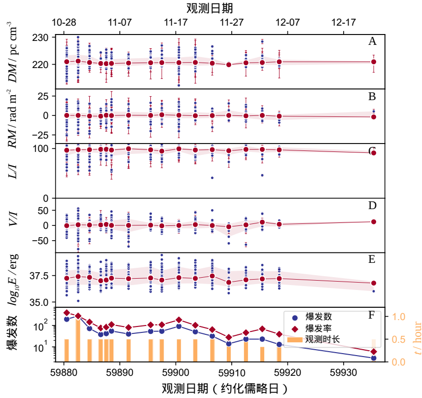
图9 FRB 20220912A 的 DM、RM、线偏振度、圆偏振度、能量、爆发率分布图 (2022 年 10 月 28 日至 2022 年 12 月 22 日 FAST 的观测) [26] 。
