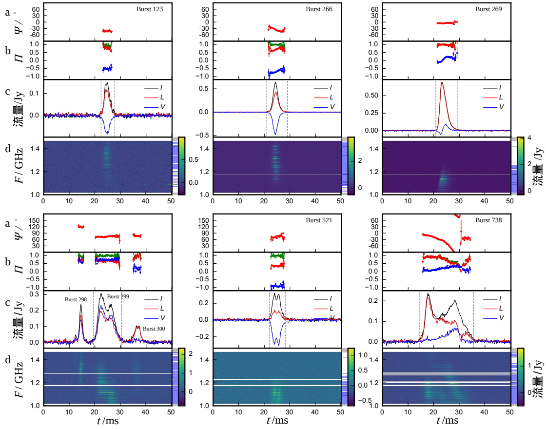
图 2 Jiang 等报告的 FAST 观测 FRB 20201124A 数据中具有高圆偏振度或偏振位置角突变的爆发样本的偏振测量结果。a) 偏振位置角; b) 线偏振度 (红色)、圆偏振度 (蓝色) 和总偏振度 (绿色) 作为时间的函数; c) 总强度 (黑色)、线偏振 (红色) 和圆偏振 (蓝色) 的爆发轮廓; d) 爆发的动态谱, 即强度作为时间和频率的函数, 灰色阴影表示受射频干扰和 20 MHz 频带边缘影响的被移除的频率信道, 蓝色阴影表示爆发信号出现的频率信道 [19] 。
