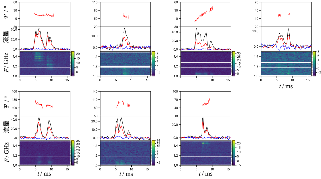
图 5 Luo 等报告的 FAST 观测 FRB 20180301A 数据中最亮的七个爆发的 PA 值、偏振轮廓和动态谱图。上图：PA 值的变化，误差棒表示 68% 置信度；中图：偏振轮廓，黑色、红色和蓝色曲线分别表示总强度、线偏振和圆偏振，流量值为归一化后的结果；底图，作为频率和时间函数的总强度的动态谱，右侧彩色条表示信噪比 [18] 。
