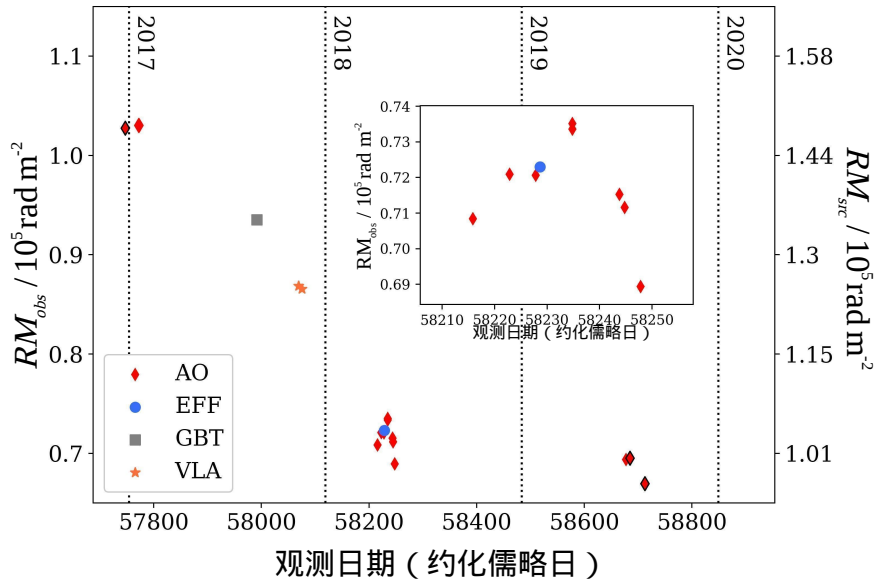
图 4 Arecibo 射电望远镜 (AO)、Effelsberg 射电望远镜 (Eff)、Green Bank 射电望远镜 (GBT) 以及甚大阵射电望远镜 (VLA) 观测的 20 个 FRB 20121102A 的 RM 值与时间的函数。 [68] 。左侧 y 轴为 RM 的观测值，右侧 y 轴为该源区域的 RM 值。
