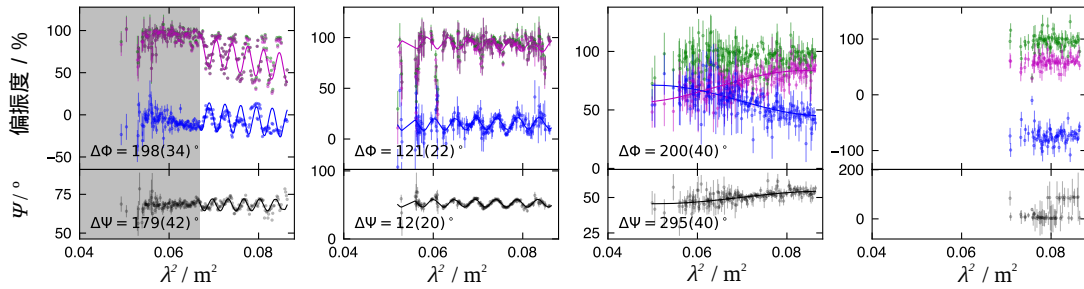
图 8 FRB 20201124A 首次发现偏振度作为波长平方的函数, 其中绿色、品红色和蓝色的点及其误差棒分别代表总偏振、线性偏振和圆偏振, 黑色代表 PA 值 [21] 。
