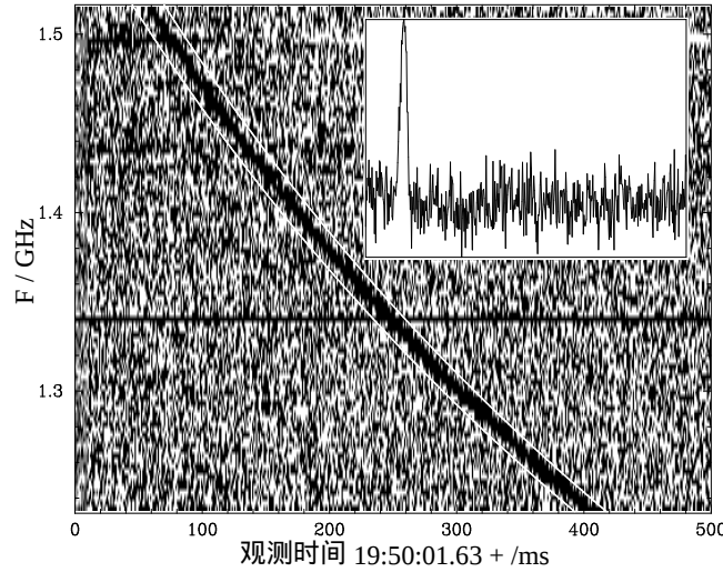
图 1 第一例快速射电暴, FRB 20010724A [3] 。
