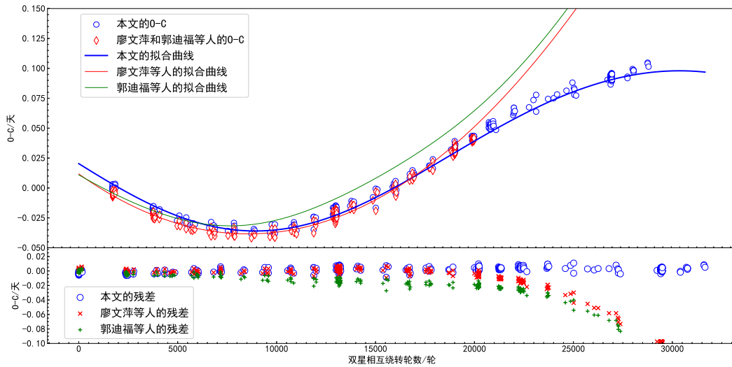
注：图中上部分为不同线性历元公式得出的 O-C 及不同研究对 O-C 的拟合曲线，下部分为不同研究对 O-C 的拟合残差。廖文萍等人 [5] 和郭迪福等人 [10] 均使用与 Vinod [4] 相同的线性历元公式，因此两次研究的 O-C 相同，但二者对 O-C 的拟合公式不同，因此拟合的曲线不一致，导致拟合后的残差（图的下部分）也有所差异。
