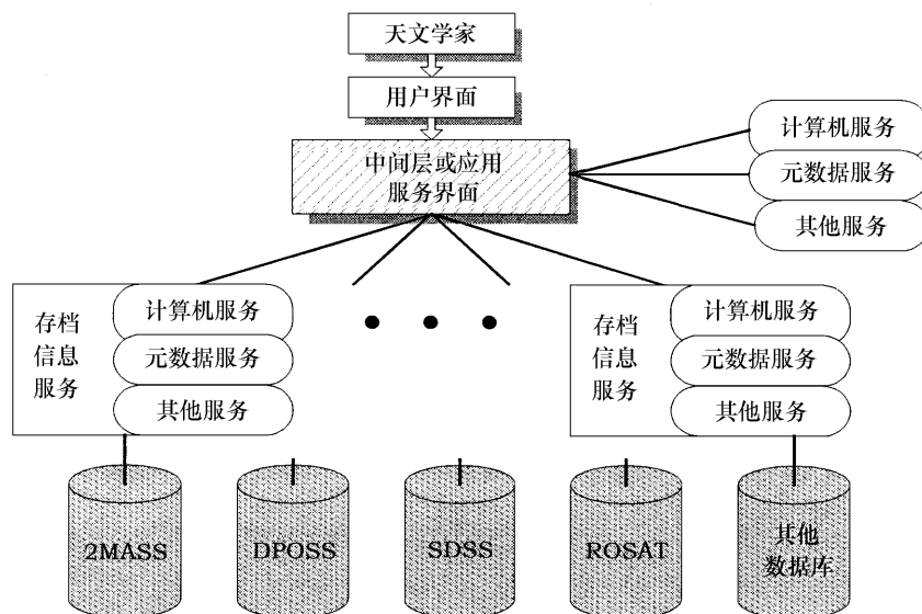
图 1 虚拟天文台结构示意图
